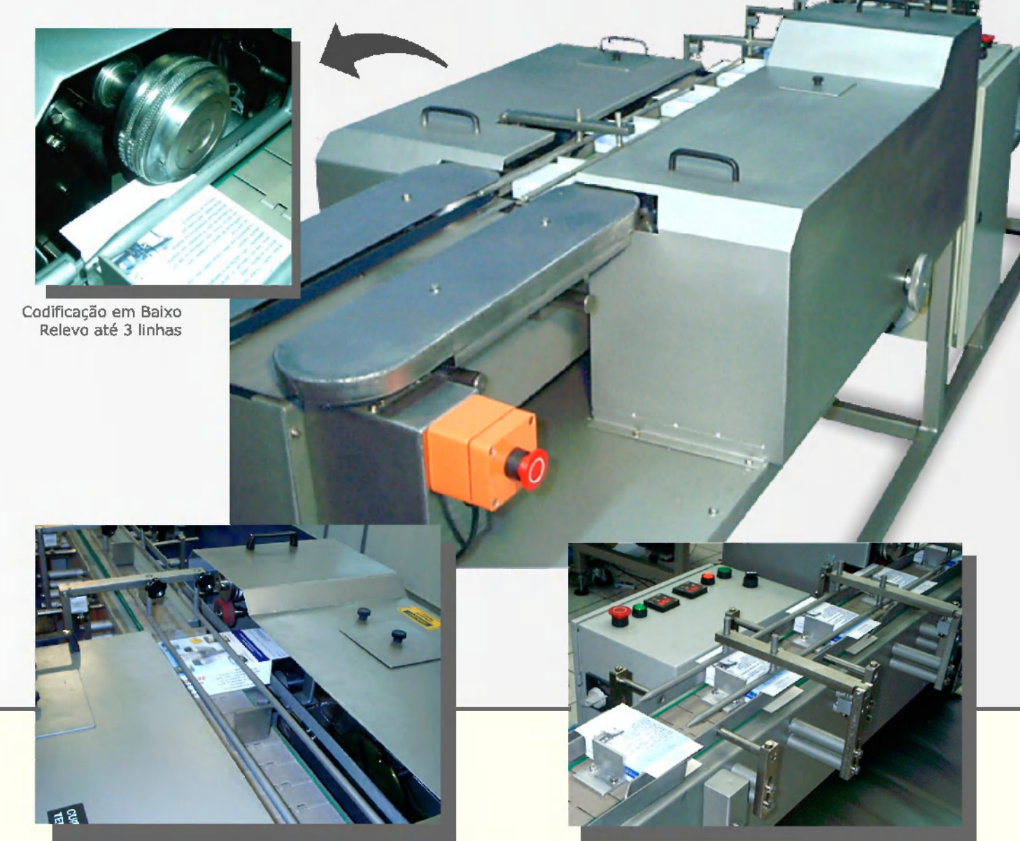
Fechadora Horizontal Contínua Modelo FHC-02
